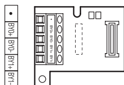
FX1N-2EYT-BD
