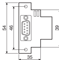
Коммуникационные адаптеры FX2N
