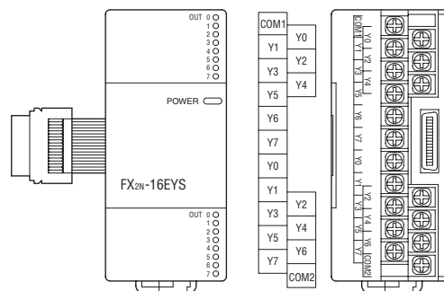
FX2N-16EYS-ES/UL
