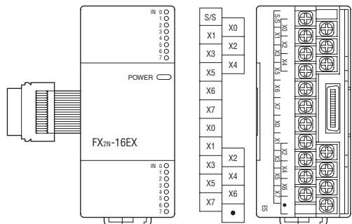
FX2N-16EX-ES/UL
