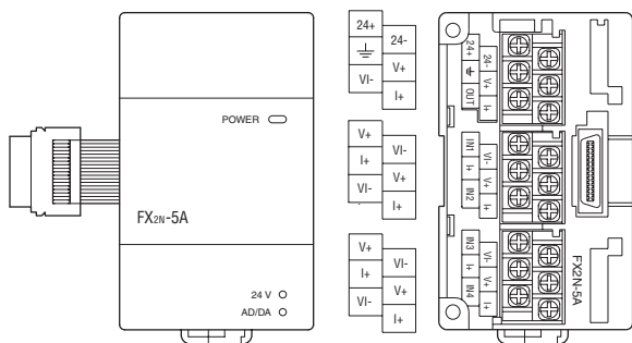
FX2N-5A
