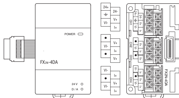
FX2N-4DA
