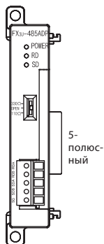
FX3U-485-ADP
