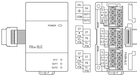
FX2N-2LC
