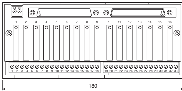
ST16-Socket
